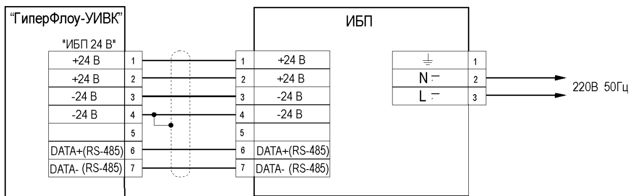
Рисунок Г.18 – Схема подключения источника бесперебойного питания ИБП-002 КРАУ4.100.002 к коммуникатору «ГиперФлоу-УИБК»
