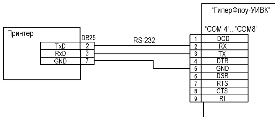
Рисунок Г.14 – Схема подключения принтера EPSON LX-300 к коммуникатору «ГиперФлоу-УИБК»
