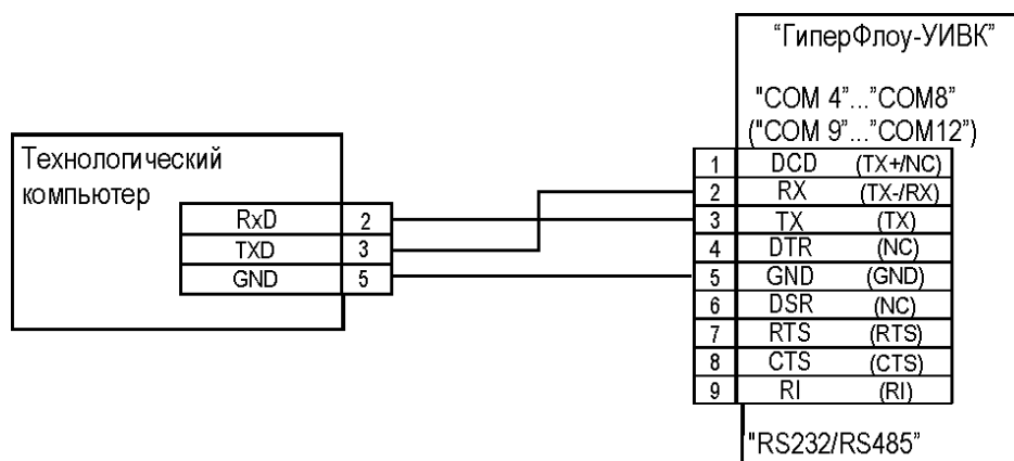
Рисунок Г.15 – Схема подключения технологического компьютера
