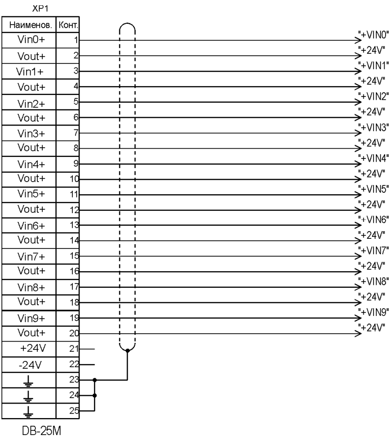
XP1 – вилка DB-25M с кожухом
