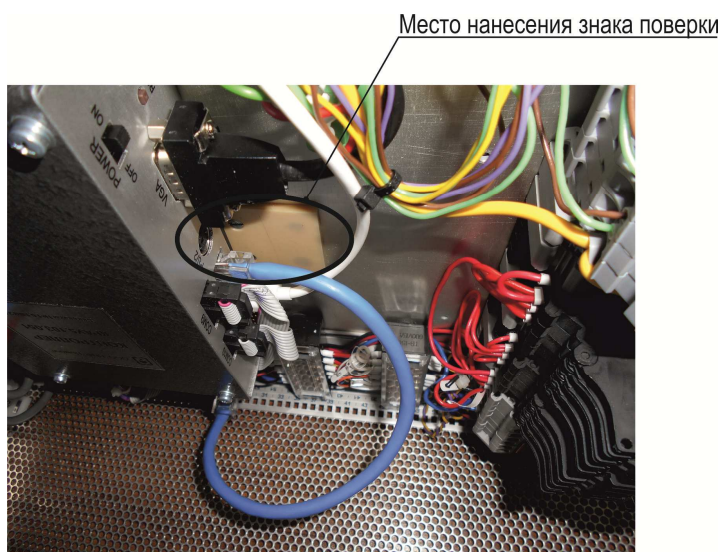
Рисунок 4 - Место нанесения знака поверки коммуникатора в крейте для монтажа в стойке 19"
