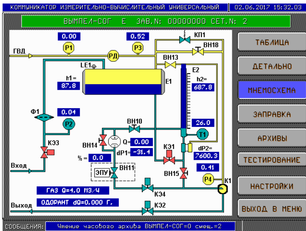
Рисунок П.32 – Мнемосхема системы «-COГ»
