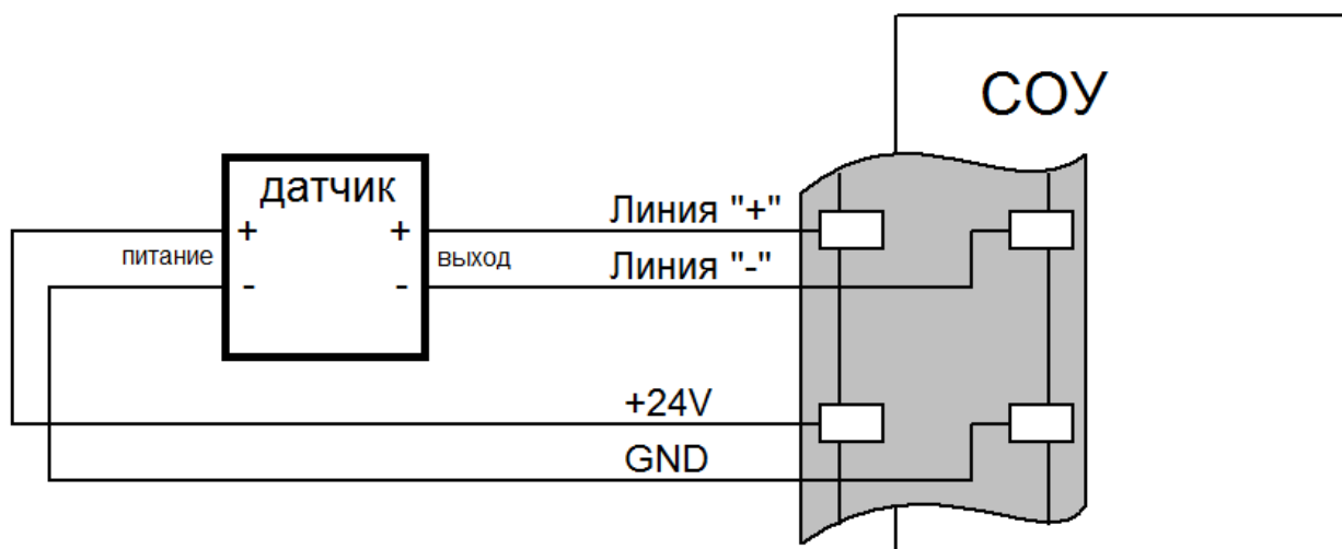
б) Подключение датчика по четырехпроводной схеме
