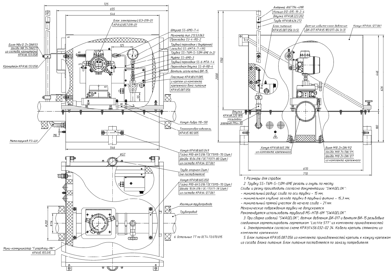
Рисунок А.4 – Вариант установки мини-коммуникатора в кожухе защитном
