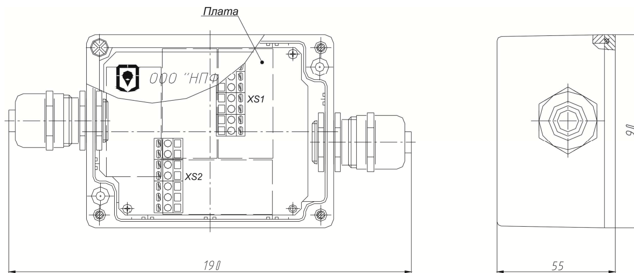
Рисунок Б.4 - Устройство управления КРАУЗ.622.075 (КРАУЗ.622.075-01)
