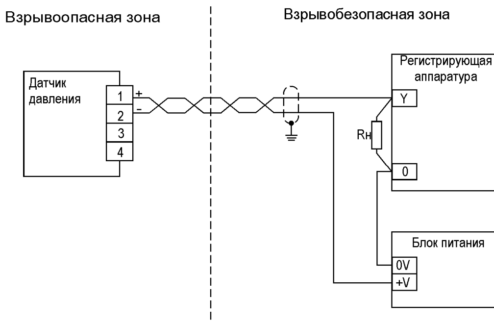
Рисунок Г.3 – Датчики с видом взрывозащиты «взрывонепроницаемая оболочка»»
